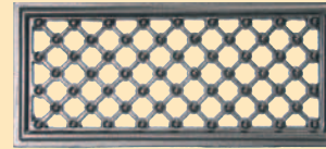
Lüftungsgitter Art. 19607: B 400 x H 180 x T 15 mm für Maueröffnung B 375 x 160 mm Aluminiumguss, lackiert, Farbe nach RAL
